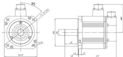
■ 中容量 中慣量SMP-M□□□20
