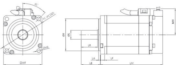
■ 小容量 低慣量SMP-L□□□30
